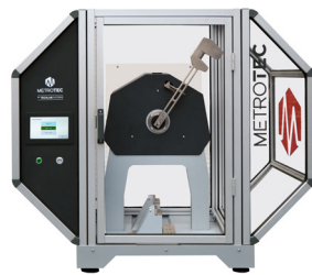
Charpy & Izod Impact Testers
